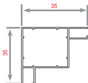
AV 22 WEIGHT 350.25 KG/M
