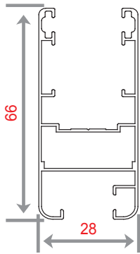
PS 6602 WEIGHT 675 .KG/M
