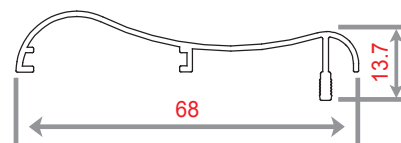
PS 9604 WEIGHT 531.19 .KG/M
