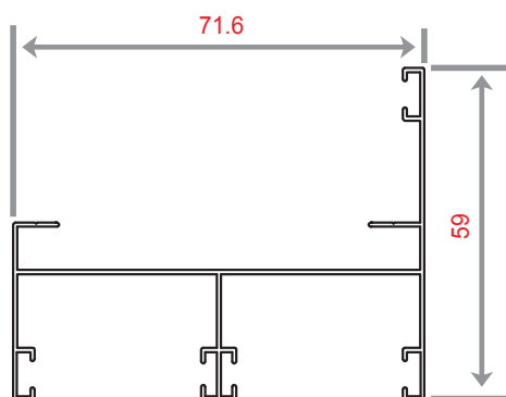
B 603 WEIGHT 630 KG/M
