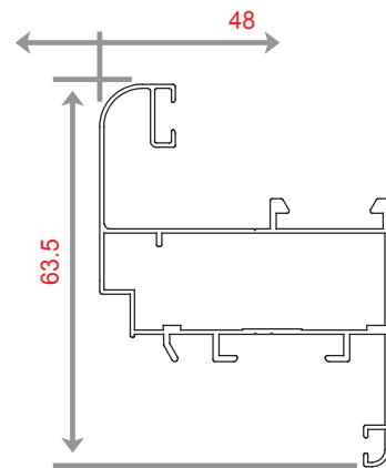
PS 4807 WEIGHT 693.33 .KG/M
