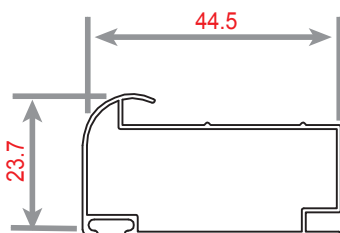
AV 26 WEIGHT 400 KG/M
