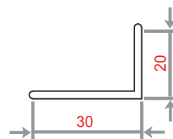
30*20*2 WEIGHT 1130.25 KG/M
