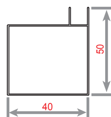
AV 35 WEIGHT 418.75 KG/M
