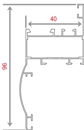
PS 4822 WEIGHT 762.3 .KG/M
