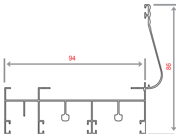
B 608-B WEIGHT 1144.8 KG/M
