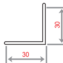
30*30*2 WEIGHT 341.99 KG/M
