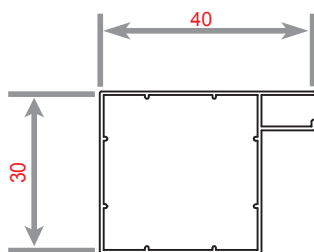
AV 28 WEIGHT 341.25 KG/M
