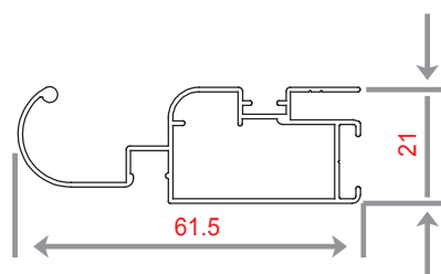
PS 9606 WEIGHT 517.88 .KG/M
