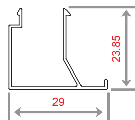
PS 5611 WEIGHT 246 .KG/M
