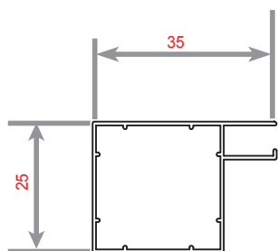
AV 01 WEIGHT 291.87 KG/M
