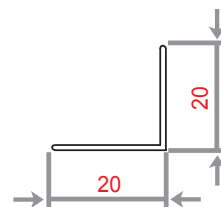
20*20*1 WEIGHT 115.22 KG/M
