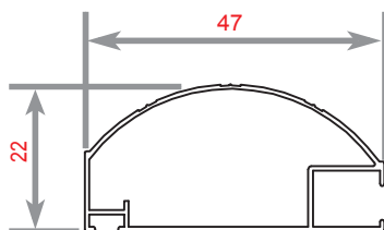
AV 08 WEIGHT 400.25 KG/M
