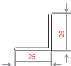
25*25*2 WEIGHT 282.48 KG/M
